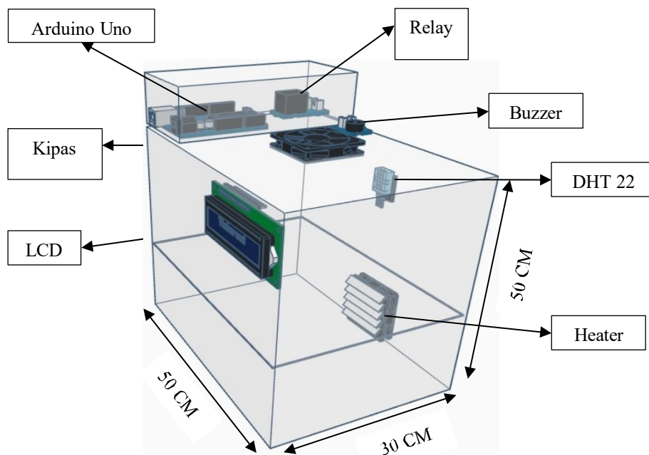
Gambar 6. Perancangan Alat
