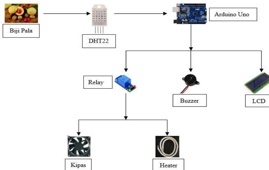
Gambar 3. Arsitektur Sistem
